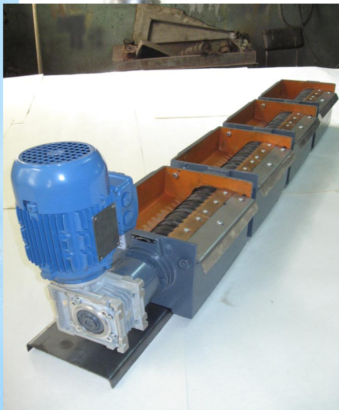
Сепаратор магнитный модели Х43-43...-47
